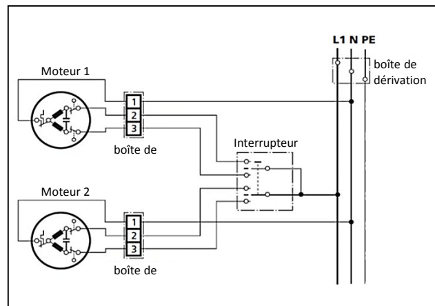
Câblage avec interrupteur bipolaire
